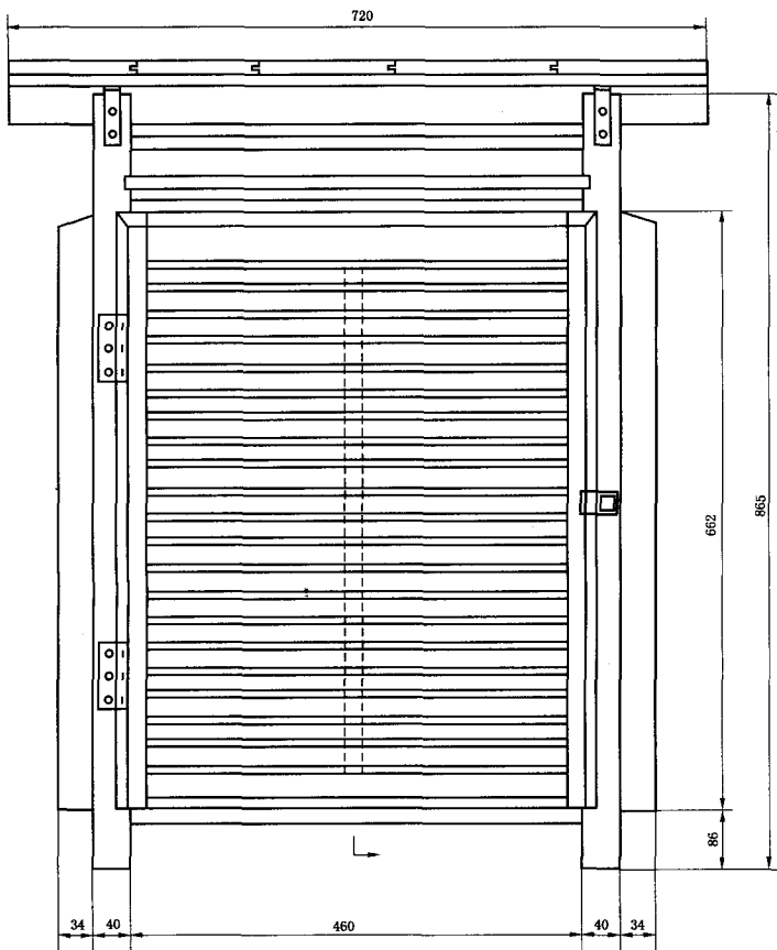
图3 大百叶箱正面图
